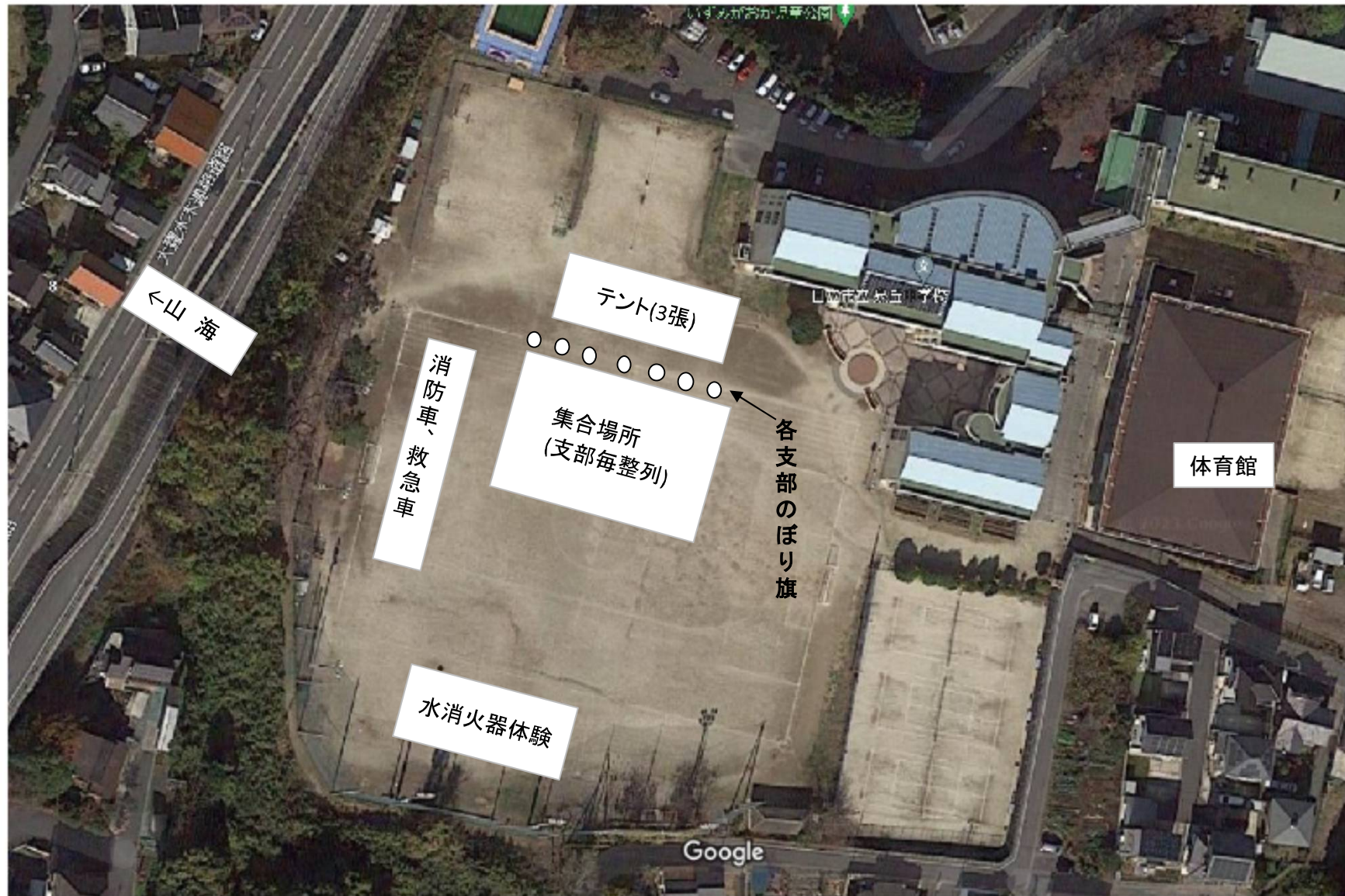
総合防災訓練会場(泉丘中学校)配置図
